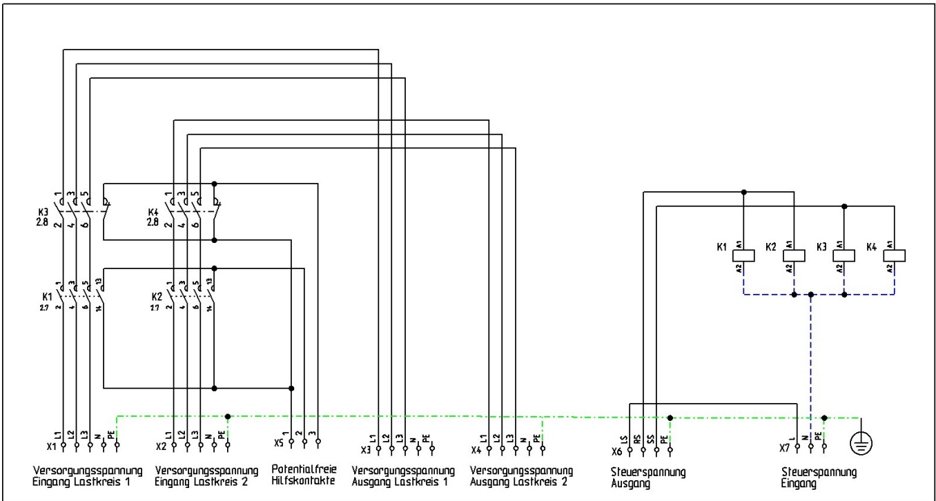
Schützkasten Extern Typ 3 und 4
